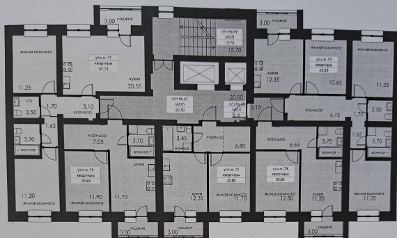
План 2 этажа 3 секция
